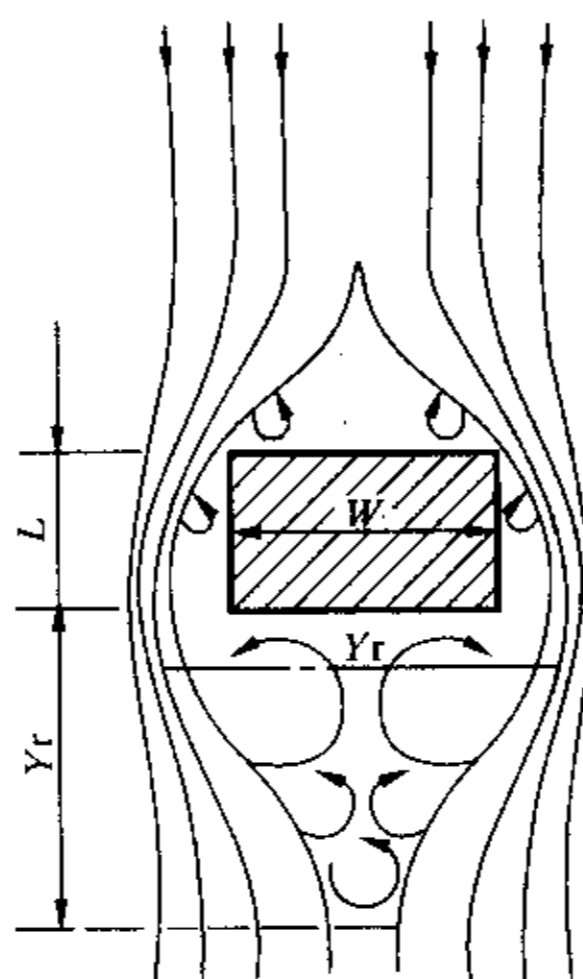
图 2 孔穴尺寸估算示意
