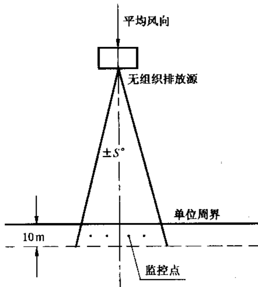
图3 一般情况下的监控点设置示意图
