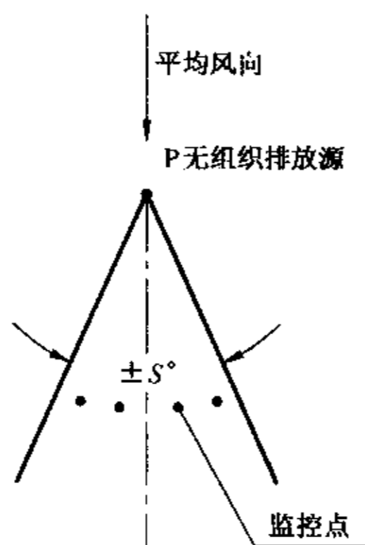
图 8 一般情况下设置监控点的方法
