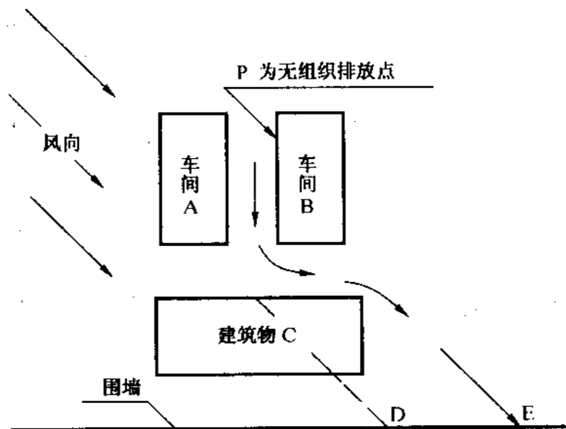
图5 局地流场分析和监控点设置示意图
