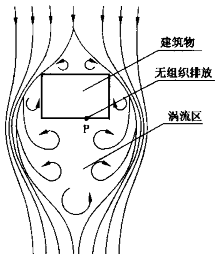
图 9 无组织排放的污染物处于涡流区内
