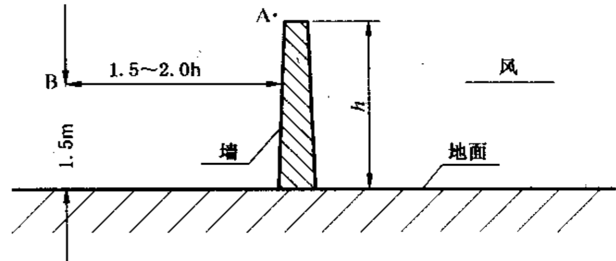
图4 不透风围墙外设监控点的参考方法
