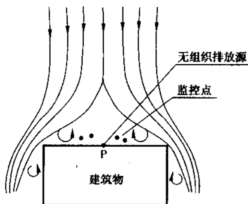
图 11 排放源处于正迎风面的监控点设置
